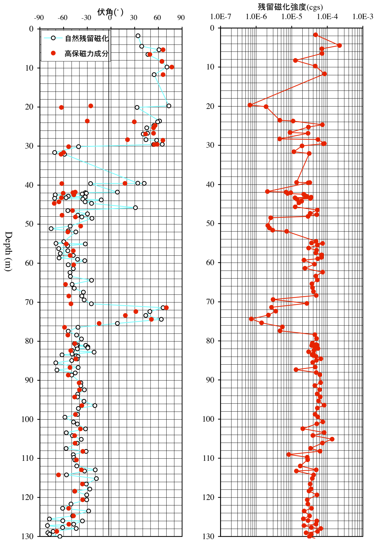
自然残留磁化測定結果解析綜合柱状図
